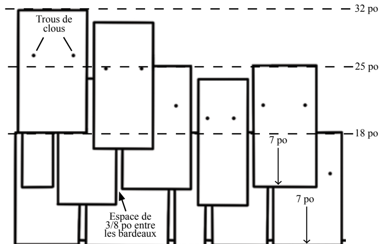
Pose de rangs décalés d'ardoises DaVinci avec un pureau de 7 po (selon la pente, les tuiles peuvent également être posées avec un pureau de 6 po)
